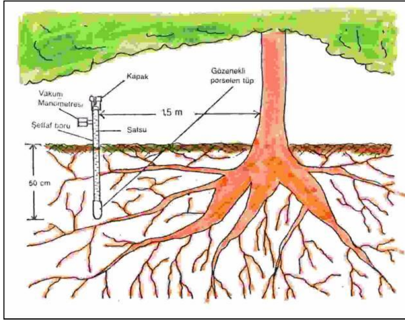
Şekil 25. Tansiyometrenin bahçeye yerleştirilmesi
